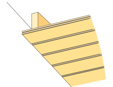
Takpanelen spikas eller skruvas i varje regel.
