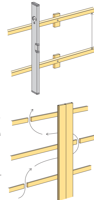
Spikläkt för ventilerad panel.
