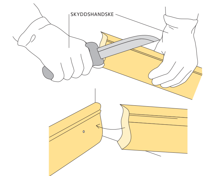
STUMFOG/SKARV INNERHÖRN
