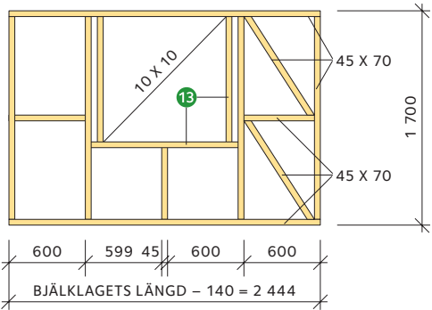
REGELSTOMME FÖNSTERGAVEL
