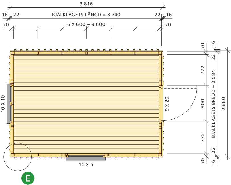
TAKSTOLSRITNING
