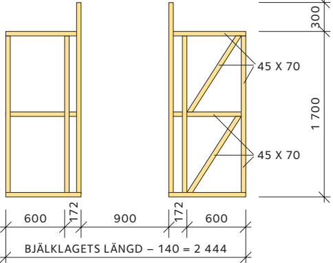
REGELSTOMME DÖRRGAVEL
