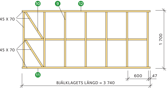
REGELSTOMME LÅNGSIDA
