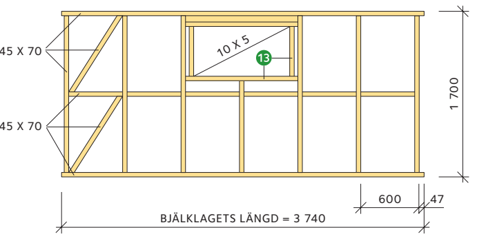
REGELSTOMME LÅNGSIDA/FÖNSTER
